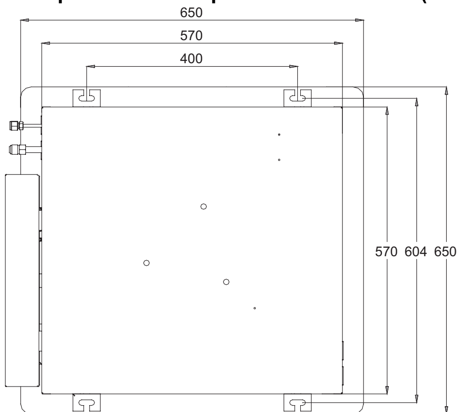
Obr. 2. Rozměry pro instalaci
