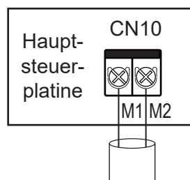
Verbindung zu ODU M1M2 (HyperLink)
