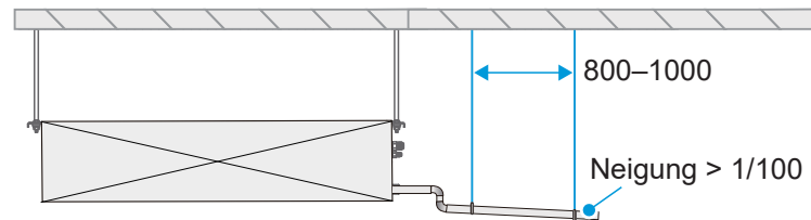
Methode zum Anschluss des Abflussrohrs für eine einzelne Einheit
