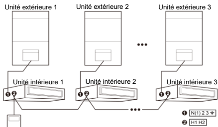
Fig. 4.6: Un panneau de commande mural commande plusieurs unités intérieures UNI SPLIT à la fois
