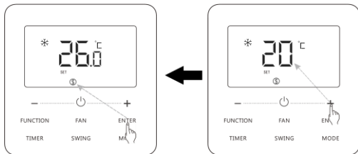
Fig. 5.4: Configuration de la fonction Basse consommation d'énergie en mode Climatisation
