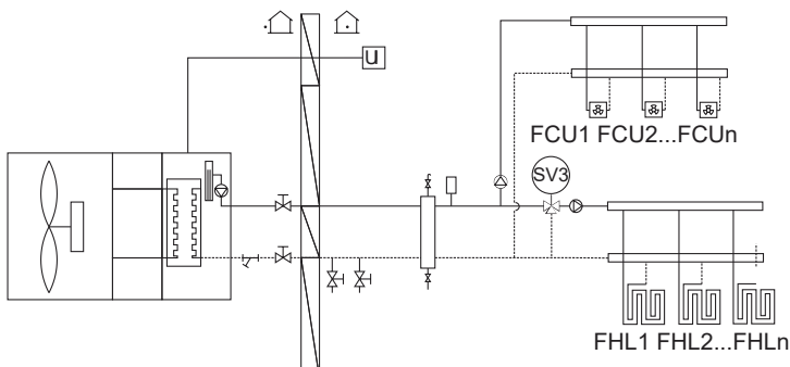
Schema dell'impianto 3
