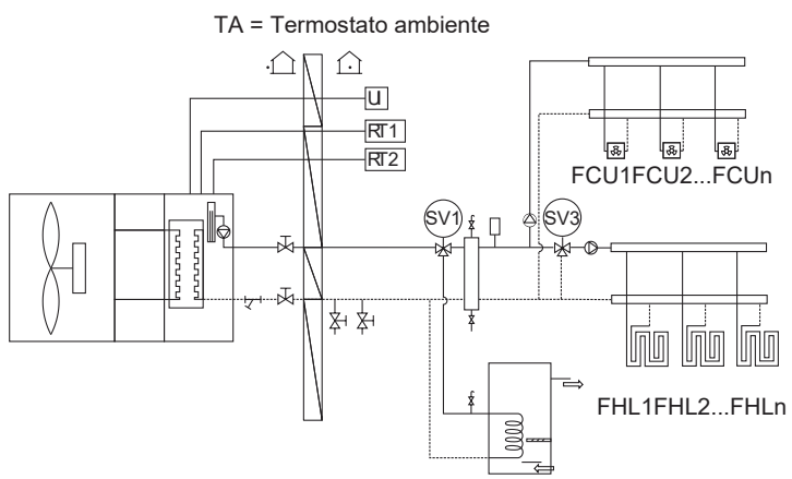
Schema dell'impianto 4
