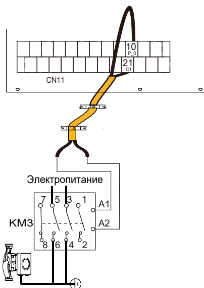
наружный циркуляционный насос P_o
