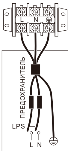
ПИТАНИЕ БЛОКА 1-фазное
