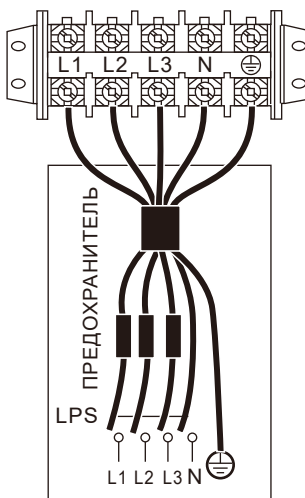
ПИТАНИЕ БЛОКА 3-фазное
